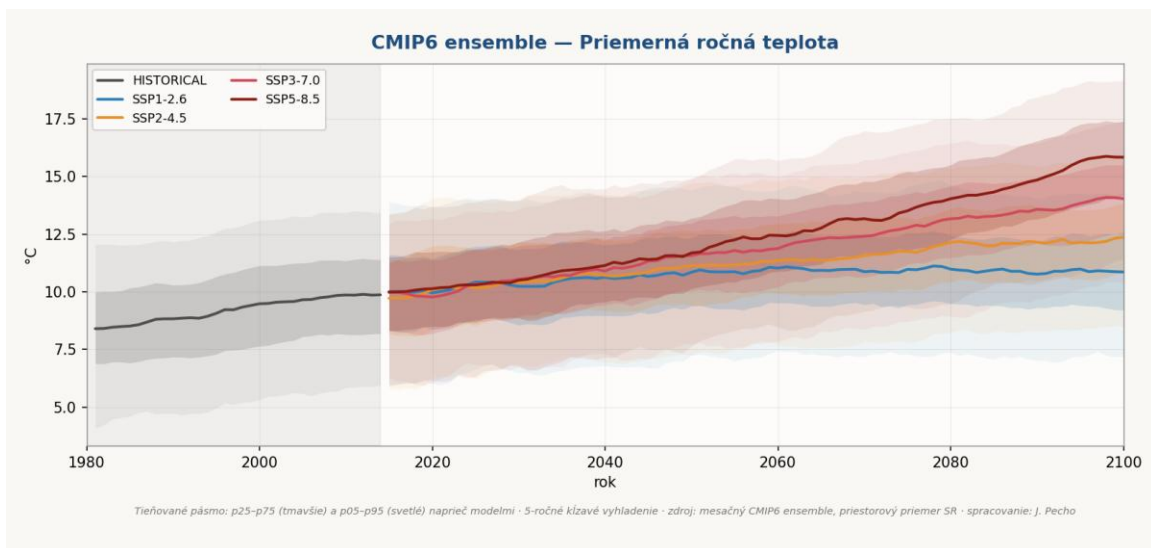
Obr. 5 Vývoj priemernej ročnej teploty pre štyri scenáre SSP; pásmo = rozpätie ansámblu. Zdroj: CMIP6 ansámbl.
