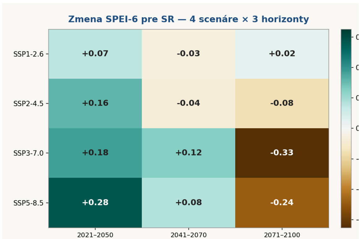
Obr. 11 Matica zmeny SPEI-6 pre SR — 4 scenáre × 3 horizonty; hnedá = posun k suchším podmienkam. Zdroj: CMIP6 ansámbel, národný priemer.
