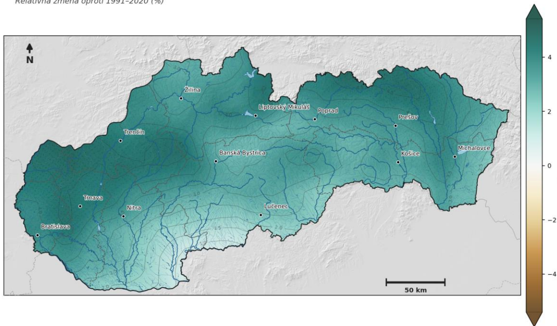
Obr. 3 Relatívna zmena ročného úhrnu zrážok (%) — SSP2-4.5. Zdroj: CMIP6 ansámbl (medián), 1 km.
