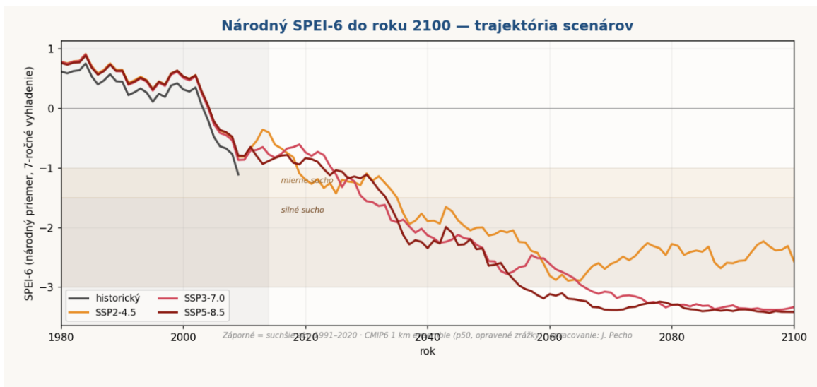
Obr. 9 Národná trajektória indexu SPEI-6 do roku 2100; vodorovné pásy označujú prahy mierneho a silného sucha, záporné hodnoty = suchšie. Zdroj: CMIP6 1 km ansámbl (medián).
