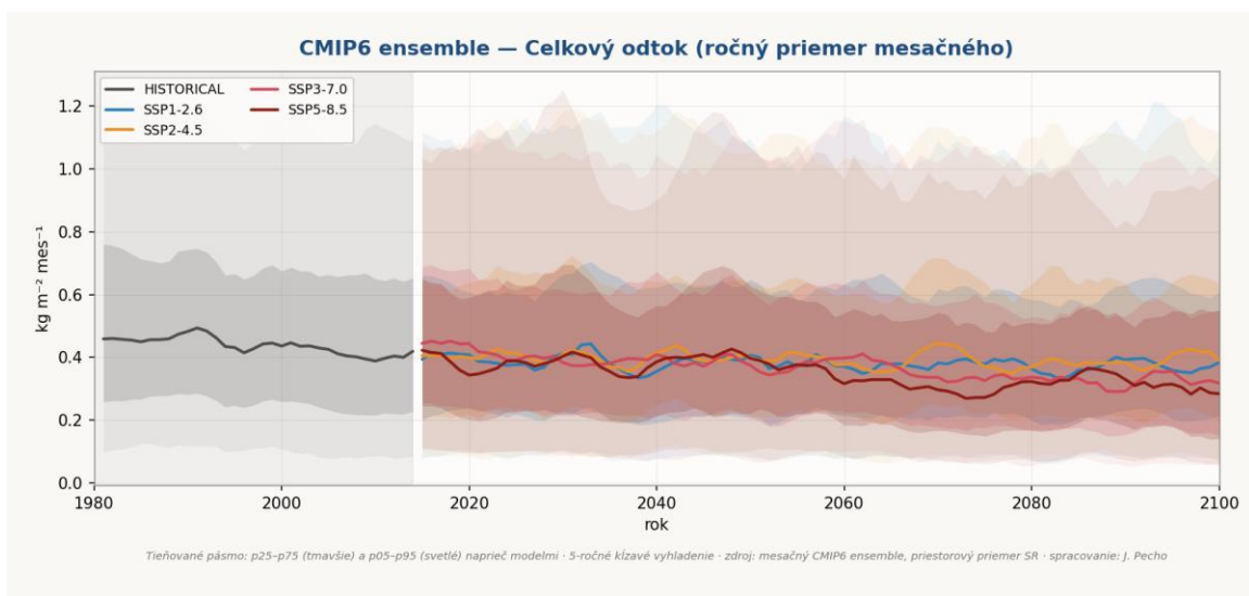
Obr. 8 Vývoj celkového odtoku pre štyri scenáre SSP. Zdroj: CMIP6 ansámbl.
